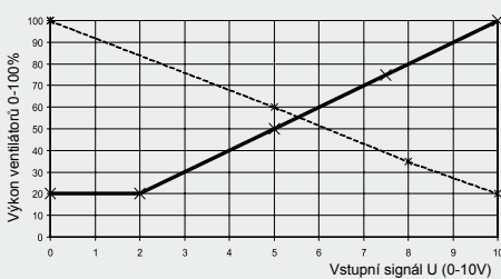
Obrázek 22 – převodní křivka OXA
