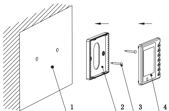
Obr. 8: Schéma instalace
